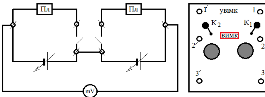
Рис. 4. Схема для дослідження послідовного з'єднання сонячних батарей
