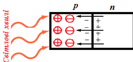
Рис. 2. Схематичне зображення процесу утворення фото-ерс
