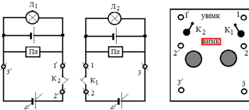
Рис. 3. Схема для вивчення дослідної установки
