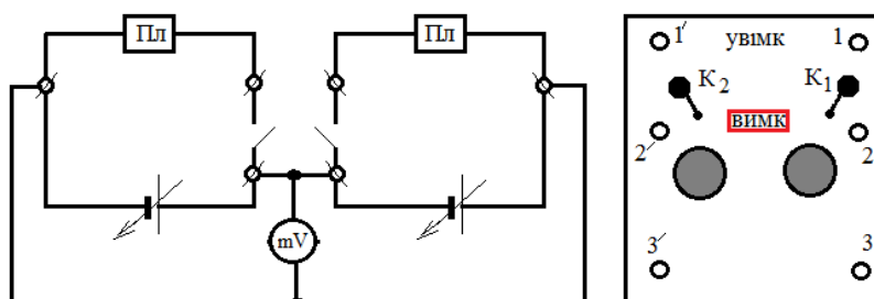
Рис. 5. Схема для дослідження паралельного з'єднання сонячних батарей
