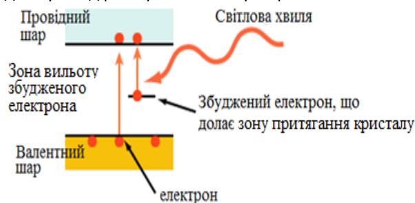
Рис. 1. Схема пояснення механізму утворення внутрішнього фотоелектричного ефекту
